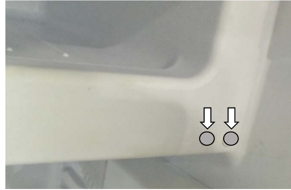
Plastik Blindstopfen rechts einsetzen Fix the plugs to the opposite/right side
